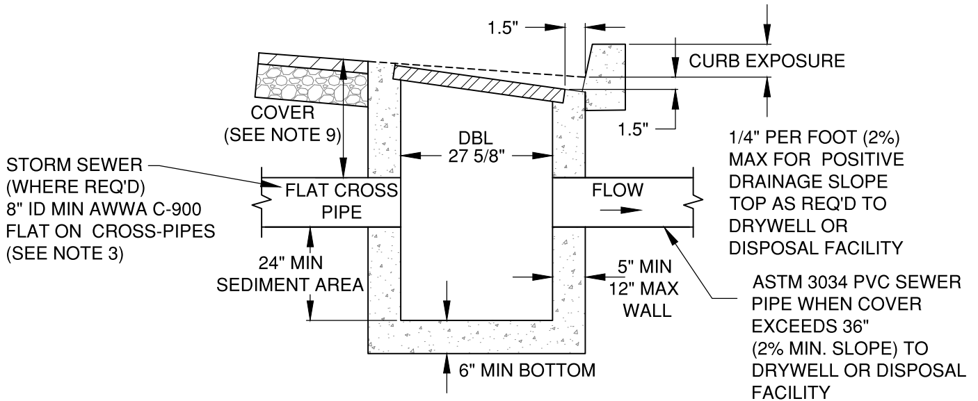
SECTION A-A
